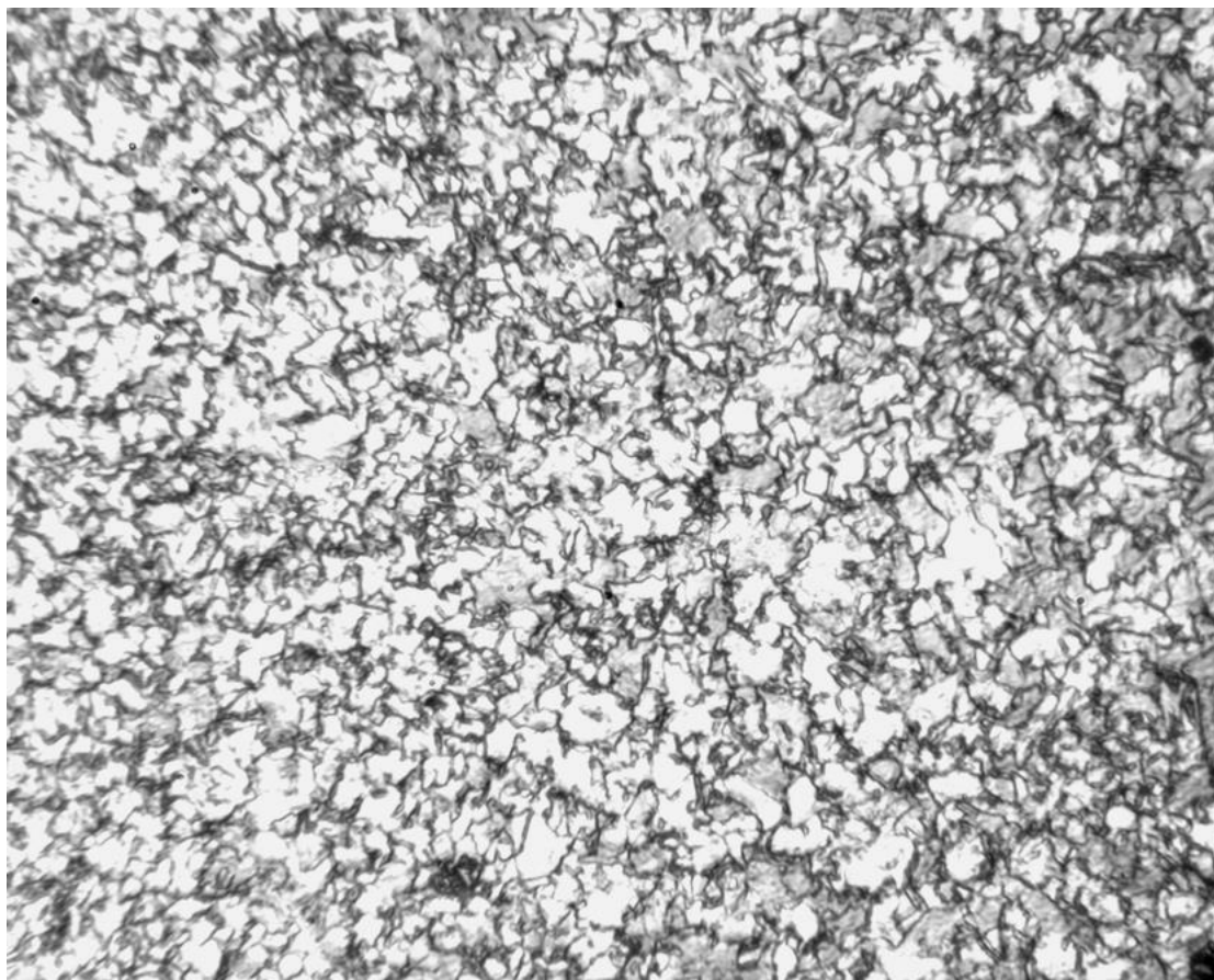
图 2. 现场金相图谱，部件名称：再热热段管道，材料牌号：12Cr1MoVG，热处理状态：退火，金相侵蚀剂：4%硝酸酒精，金相组织：粒状贝氏体+少量碳化物，放大倍率：400 倍
