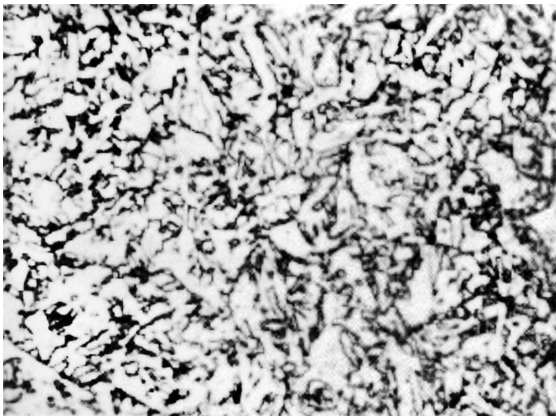
图 3. 现场金相图谱，部件名称：板材，材料牌号：12Cr1MoV，热处理状态：980℃正火+500℃盐浴，金相侵蚀剂：4%硝酸酒精，金相组织：粒状贝氏体，放大倍率：800 倍
