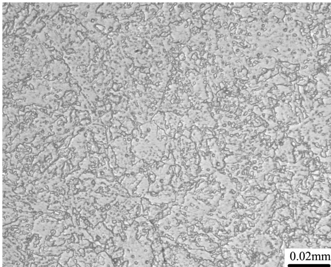
图 1.实验室金相图谱，部件名称：高温再热器出口集箱，材料牌号：12Cr1MoVG，热处理状态：正火+回火，金相侵蚀剂：4%硝酸酒精，金相组织：回火贝氏体
