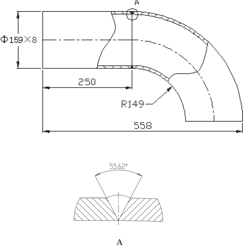
图 4 弯管段与直管段对接接头
