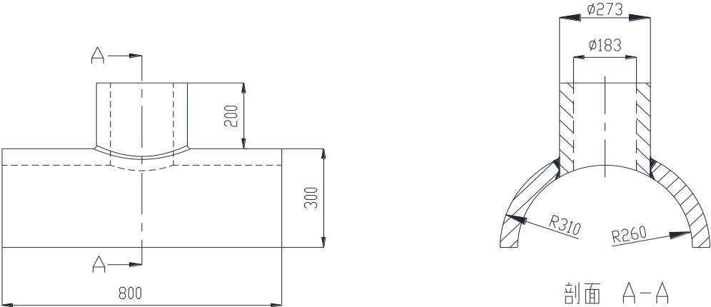
图 6 管-管插入式角接接头
