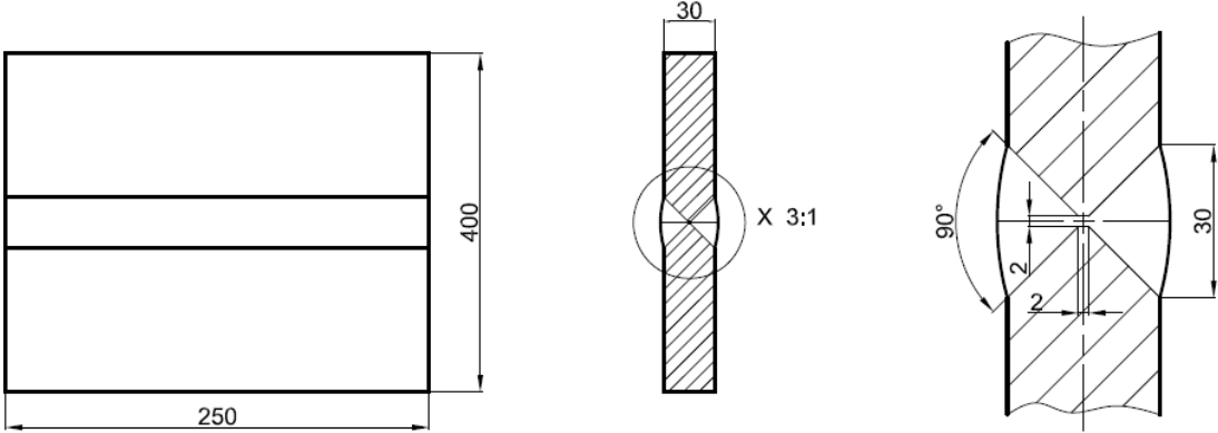
图 7 平板对接接头模拟试件
