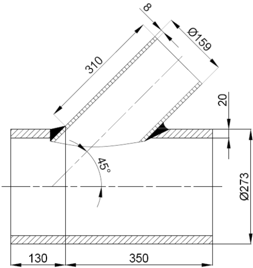
图 5 管-管斜插入式角接接头
