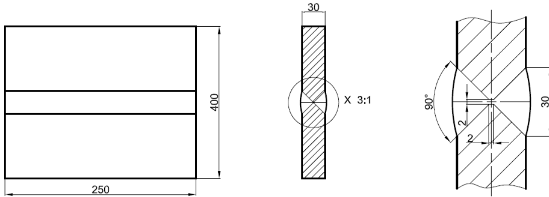
图 6 平板对接接头模拟试件
