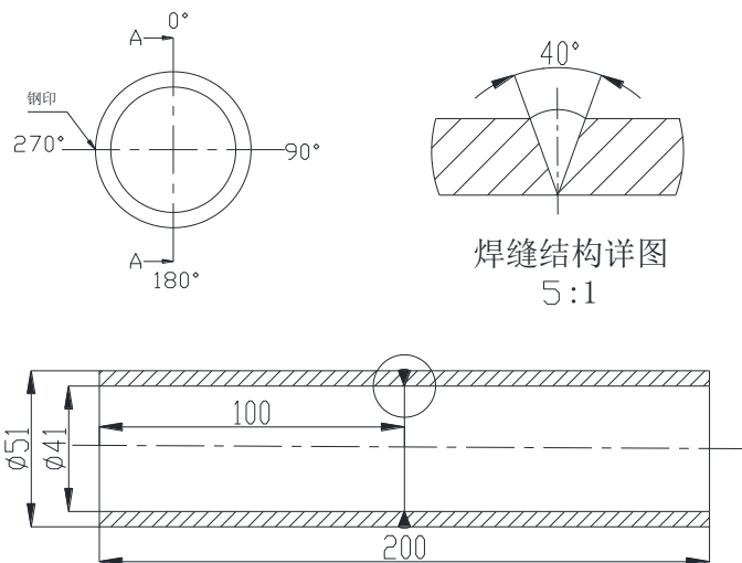
图 1 小径管对接接头
