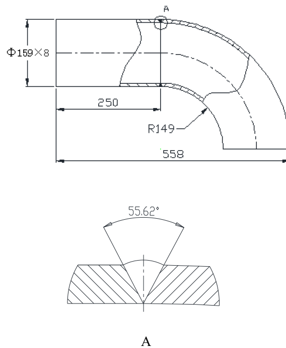
图 4 弯管段与直管段对接接头
