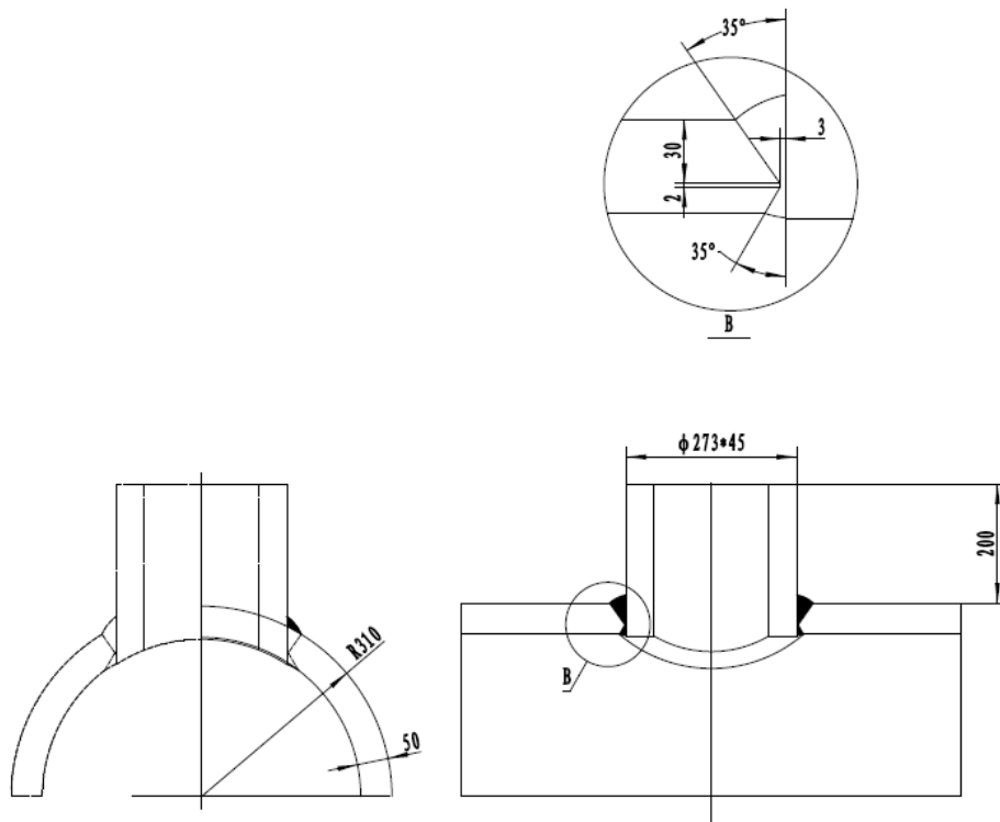
图 8 管-管插入式焊接接头模拟试件
