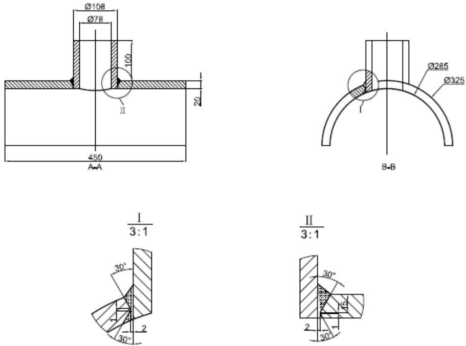
图 8 管-管插入式焊接接头模拟试件
