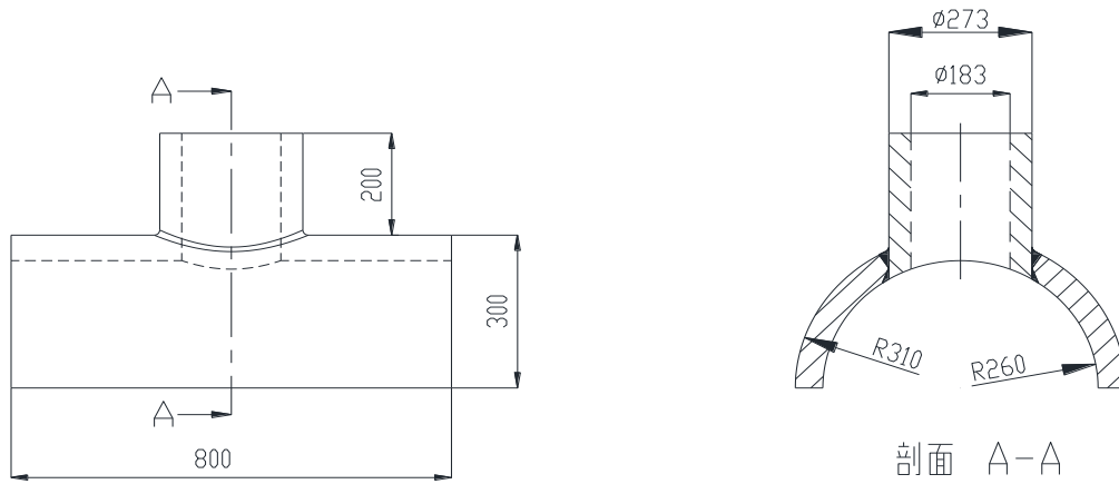
图 5 管-管插入式角接接头
