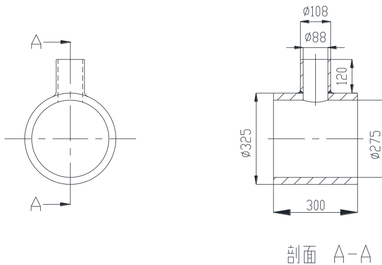
图 2 管-管安放式角接接头
