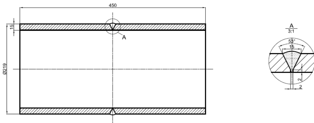
图 7 管-管对接接头模拟试件
